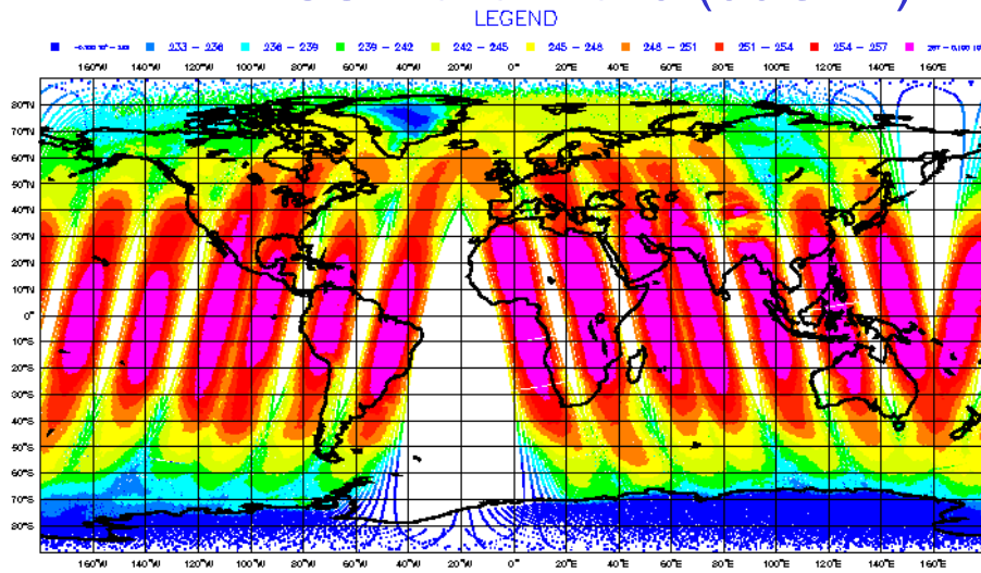
AMSUA-channel 5 (53GHz)
